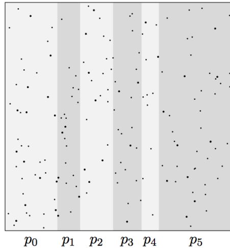
FIG. 1 – Exemple de situation initiale hétérogène, avec une distribution par bandes sur 6 processeurs, avec 112 requins et 134 sardines. (Les gros points représentent les requins, les petits les sardines.)
